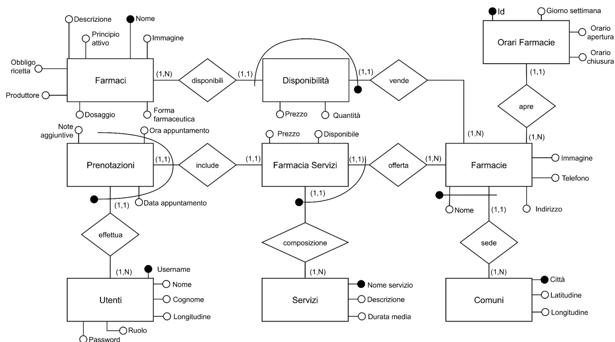
Figura 1: Diagramma ER
